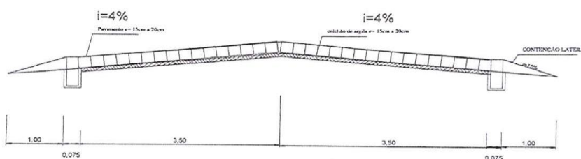
COLOCAÇÃO DAS PEDRAS IRREGULARES (DEPOIS DA COMPACTAÇÃO)
